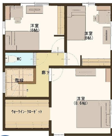
2階
